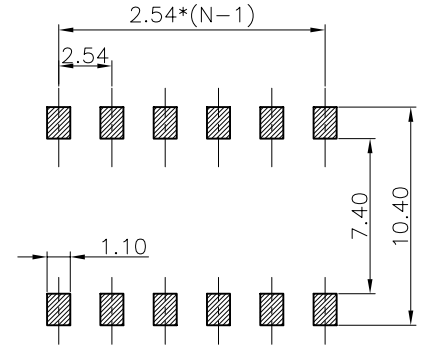
SMT TYPE
