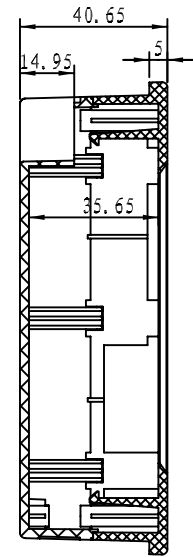
截面 A-A
