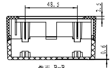
截面 B-B
